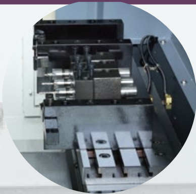
櫛式刀座 Gang type tool base
